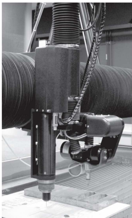
OMAX Drill Head installée à côté de la Tilt-A-Jet®
